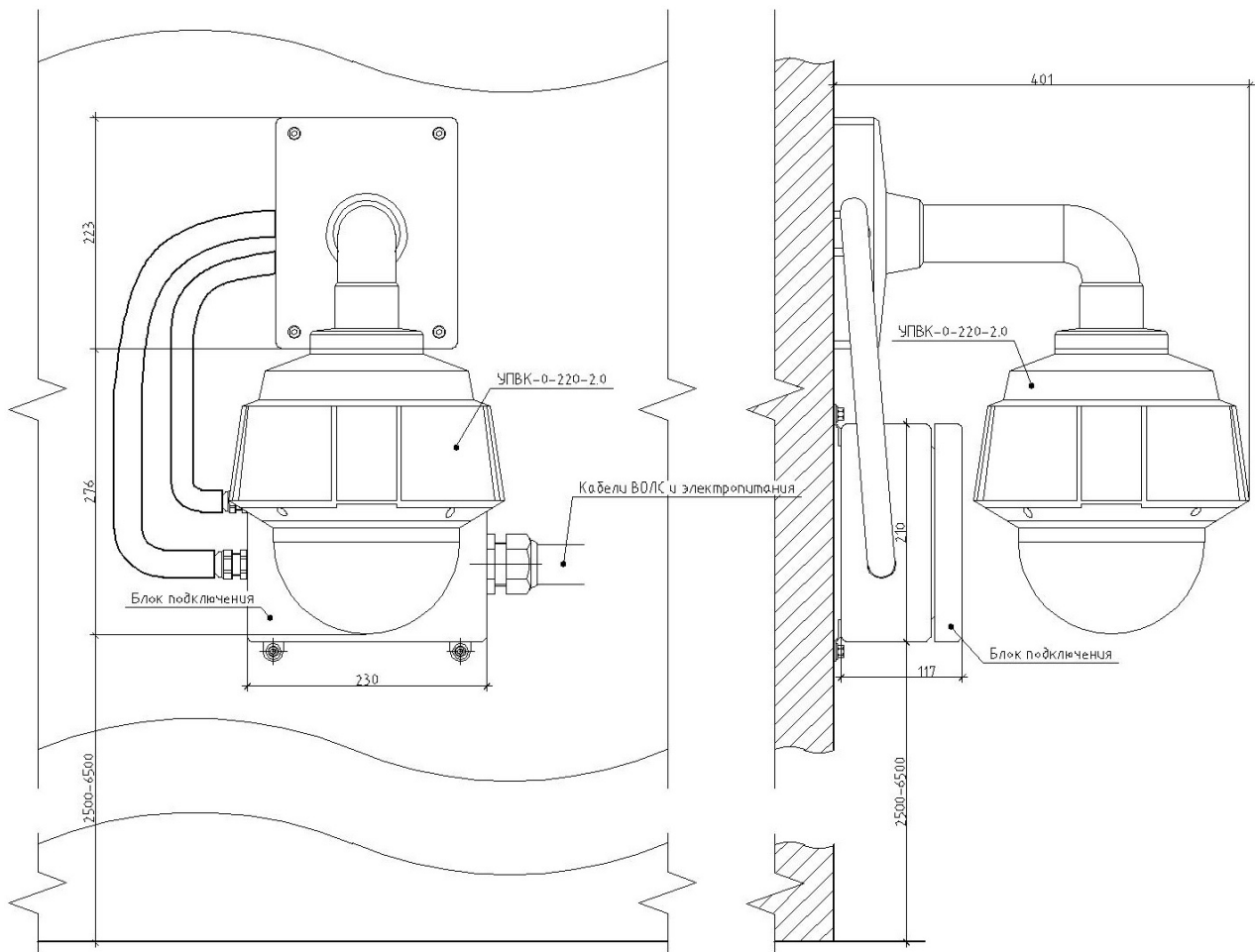
Схема установки УПК-0-220-3.0
